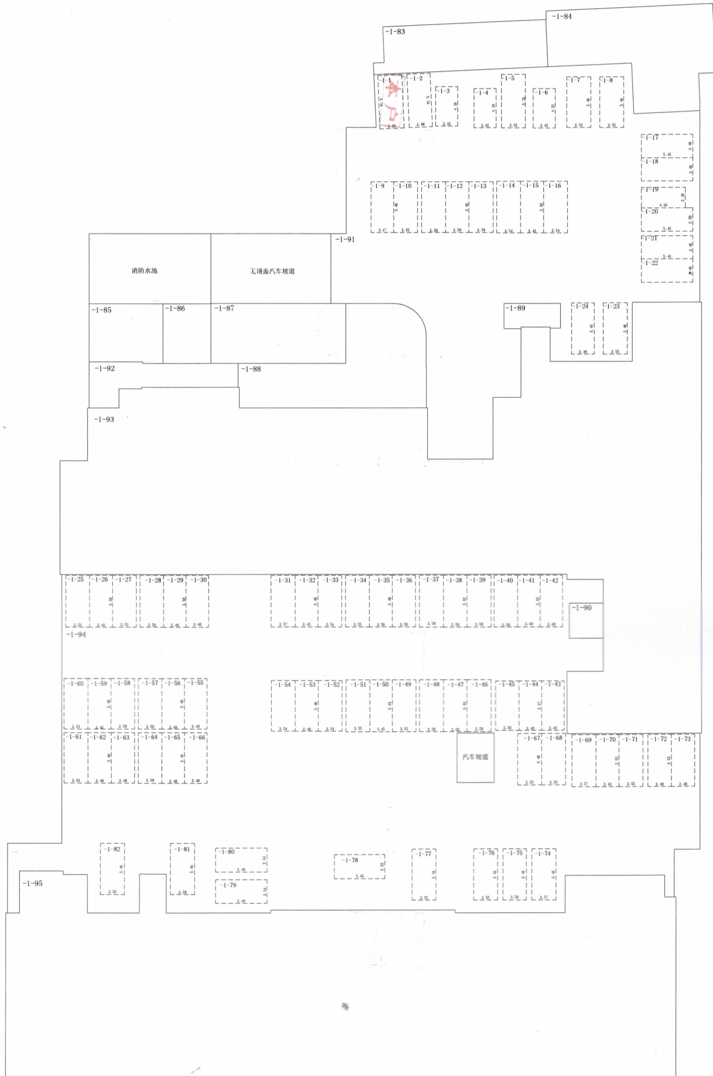
地下一层平面图
